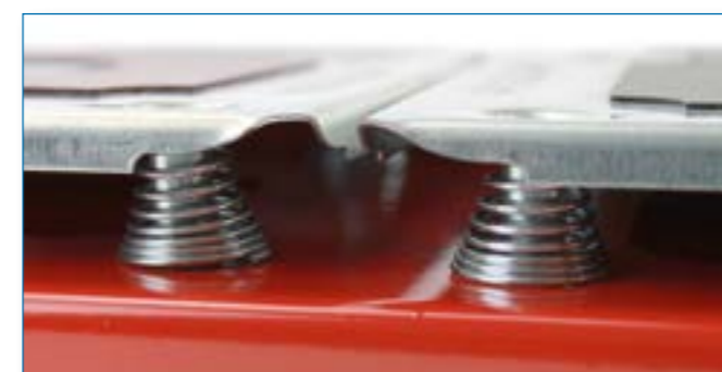
Bases sobre muelles y soprtes laterales Bases on springs and lateral supports Plateaux sur ressorts et supports latéraux
